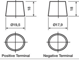
T1 Standard DIN Post
