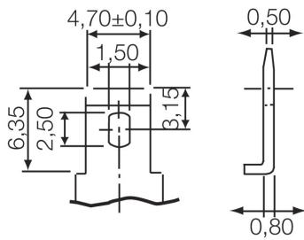
Lattaliitin 4,8 mm
