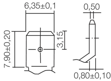
Lattaliitin 6,35 mm
