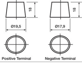
T1 Standard DIN Post
